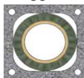
objektivHausschornstein System Einzügig
